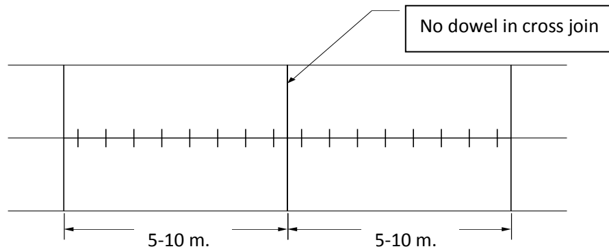
JPCP
